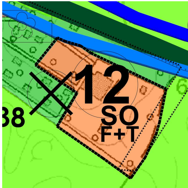
Abbildung 24: wirksamer Flächennutzungsplan
